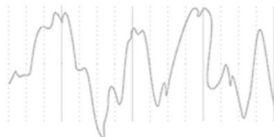
Delta (.1-3.9 Hz)
