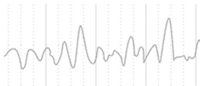
Theta (4-7.9 Hz)
